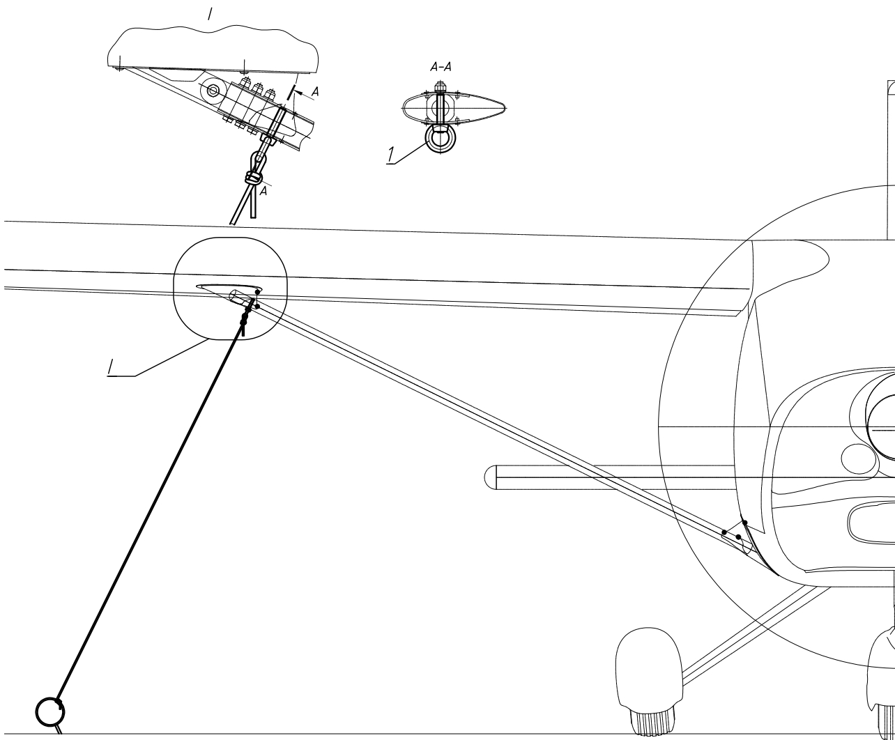
Fig. 21. Tie-down ring
